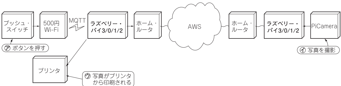
図1 モノとプリンタをリアルタイムにつなげるIoT遠隔ポラロイド的インスタント・カメラ
