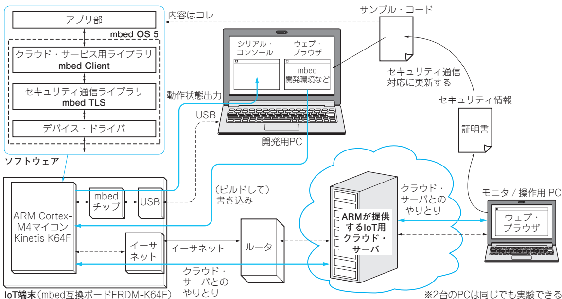
図1 ARM が提供するIoT開発ワールドを試するための実験構成
