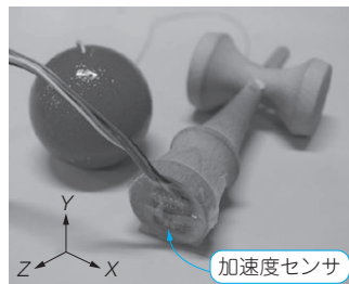
写真2 動き検出のための加速度センサをさらの部分に仕込んだ
