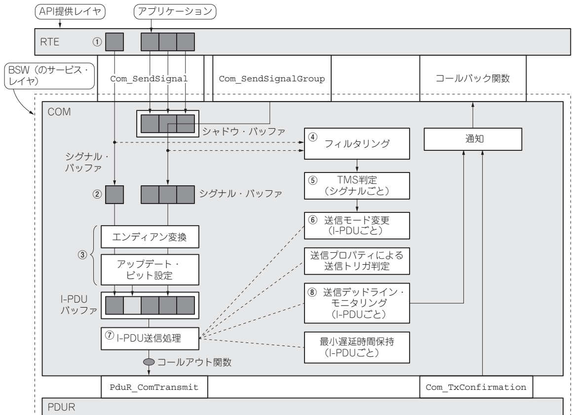
図1 COMスタックの送信モデル
