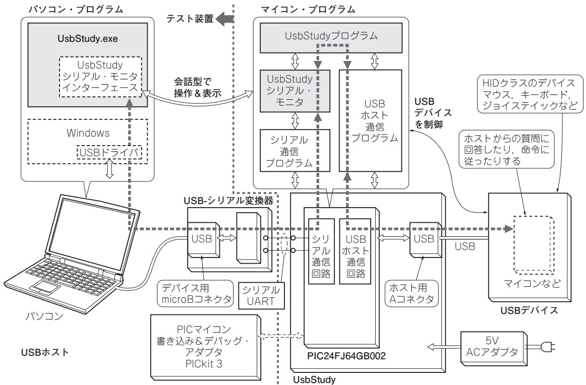
図1 USB通信ステップ・バイ・ステップ実験の構成
