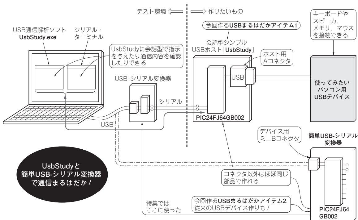
図1 本特集の実験! …USB通信をまるはだかにしてマイコンからパソコン周辺機器を動かす
