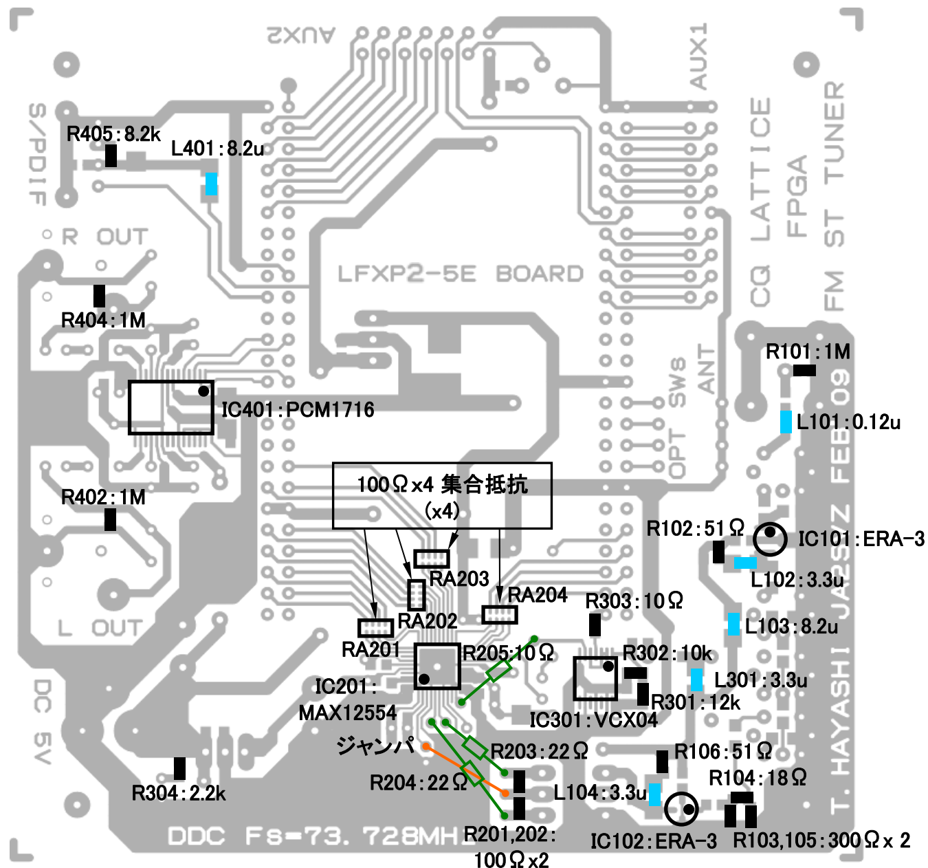
(7) 半田面:IC, 抵抗、コイルその他
