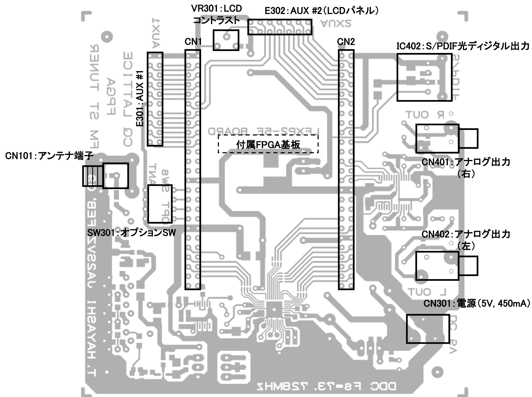
(2) 部品面:コネクタ, SW, VRの配置
